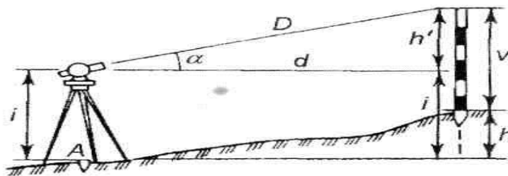
Рис. 6 Схема тригонометричного нівелювання
